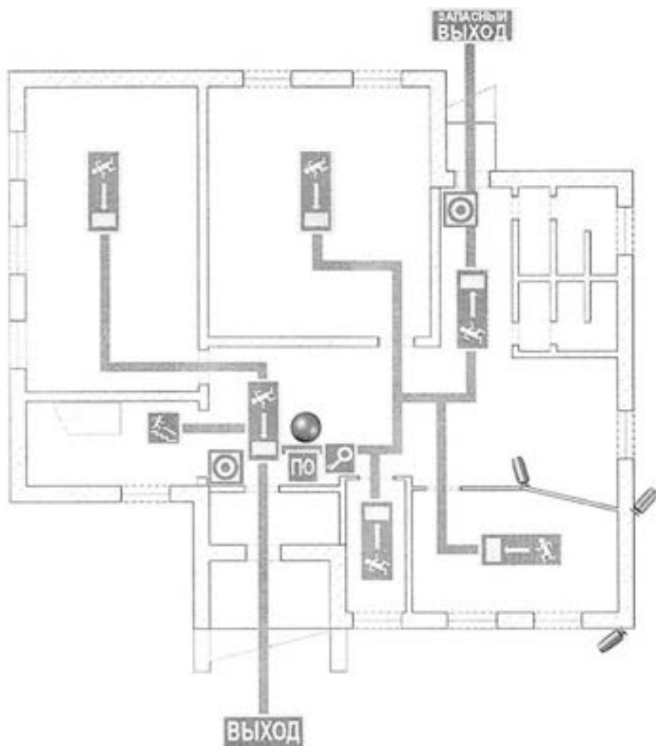
ПЛАН 1 этаж 1 корпус МАУДО "ЦДТ"
